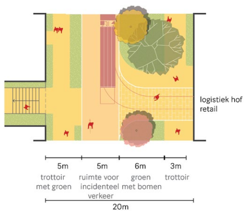
Afbeelding 63. Profielen Gemengde straat
