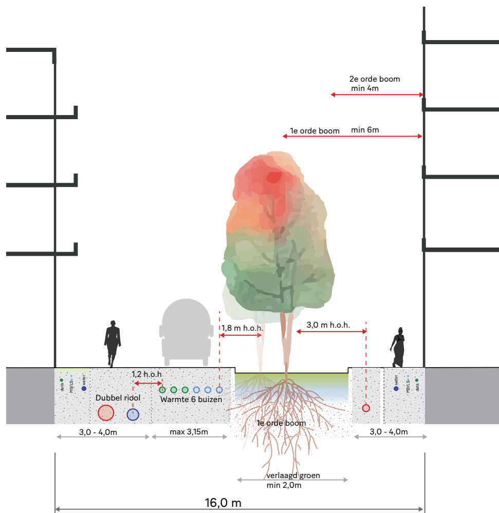
Afbeelding 197. Voorbeeld van ligging van ondergrondse infrastructuur in de straatprofiel
